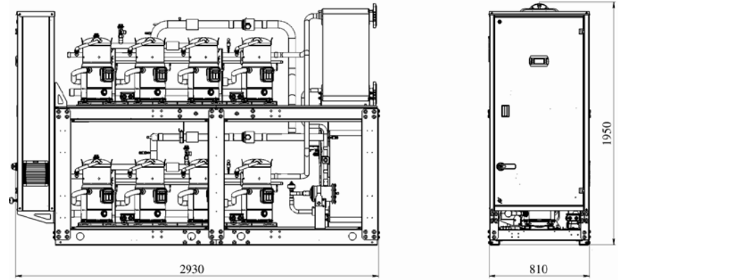
Типоразмер 510/560
