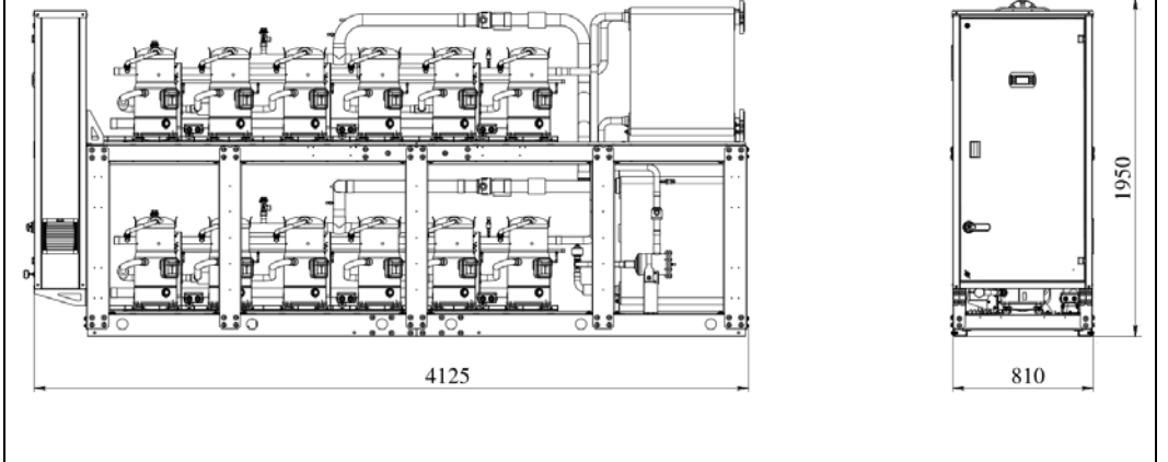
Типоразмер 760
