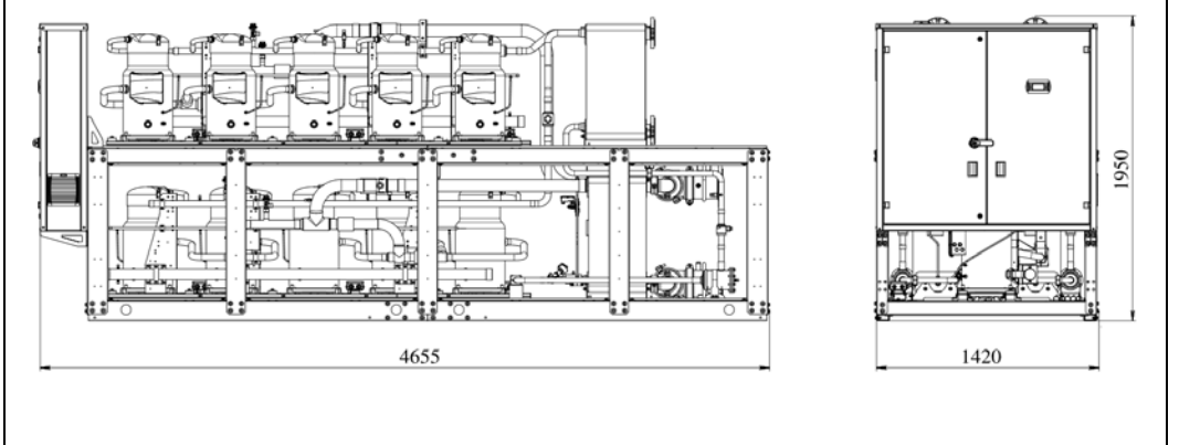
Типоразмер 900/950/1100
