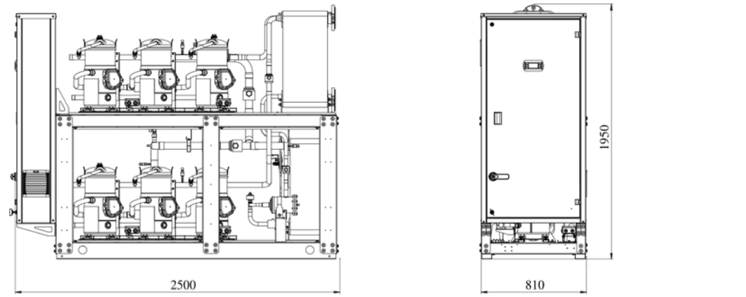
Типоразмер 380/450
