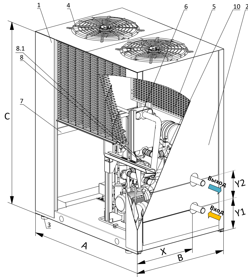
Рисунок 2.1. Основные элементы конструкции чиллеров моделей 045÷050.
