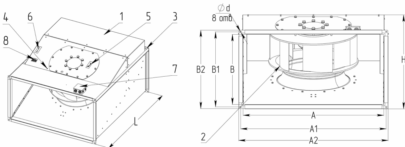
Рисунок 3.2 – Внешний вид вентиляторов VP 100-50/63.4D
