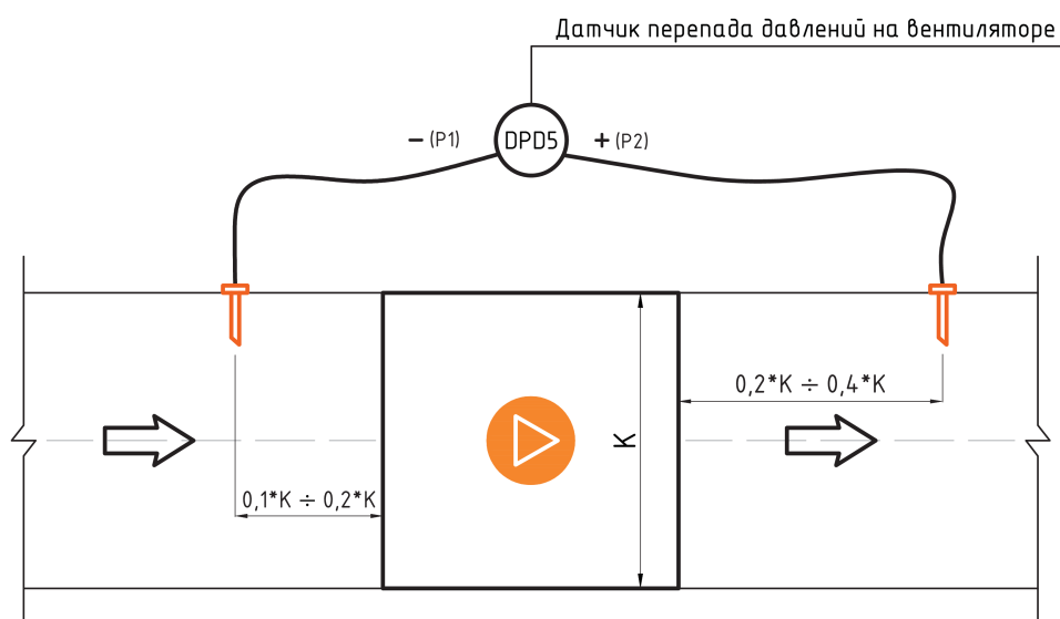
Рисунок 6.1 – Размещение датчика дифференциального давления вентилятора
