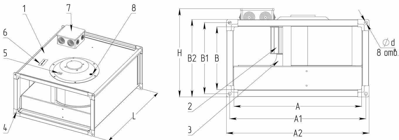
Рисунок 3.1 – Внешний вид вентиляторов VP 40-20 – 90-50
