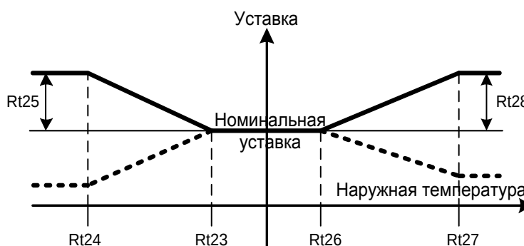
Рис.17.- Параметры компенсации уставки.
