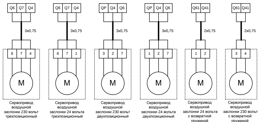
Рис. 24.- Подключение заслонок наружного воздуха.
