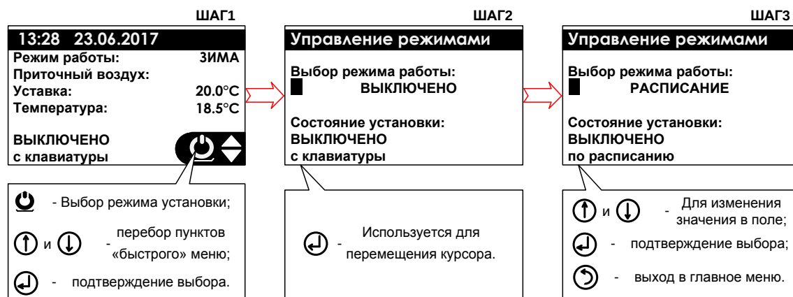
Рис 2.- Алгоритм выбора режима работы установки.
