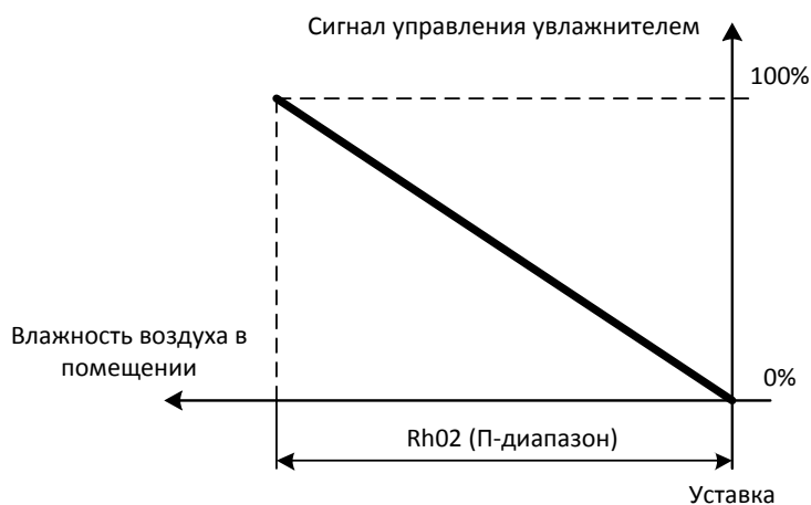
Рис.21.- Алгоритм работы парового увлажнителя.
