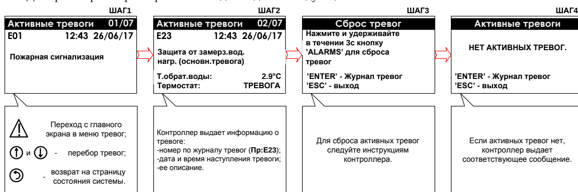
Рис.23.- Алгоритм просмотра и сброса активных тревог.
