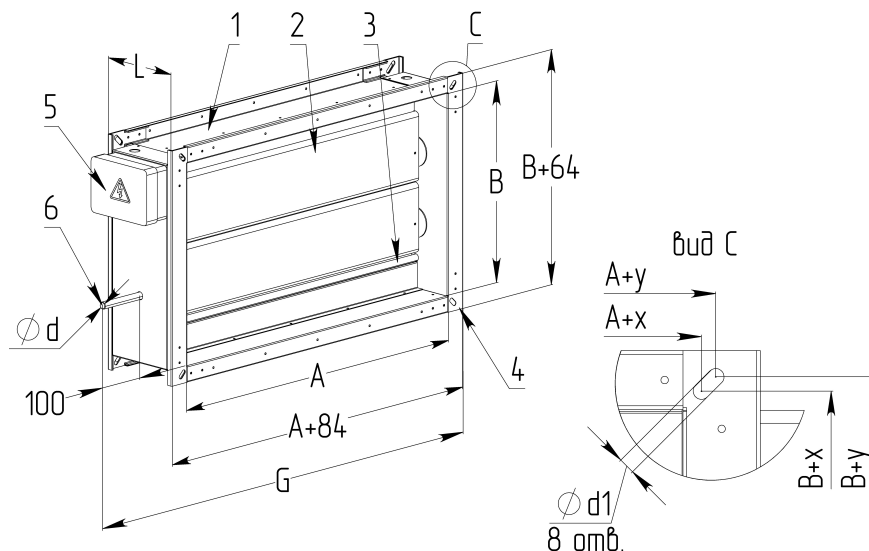
Рисунок 2.1 – Внешний вид и основные размеры заслонок 1 - корпус, 2 - лопатки, 3 - ТЭНы, 4 - фланец, 5 - распаечная коробка, 6 - шток.
