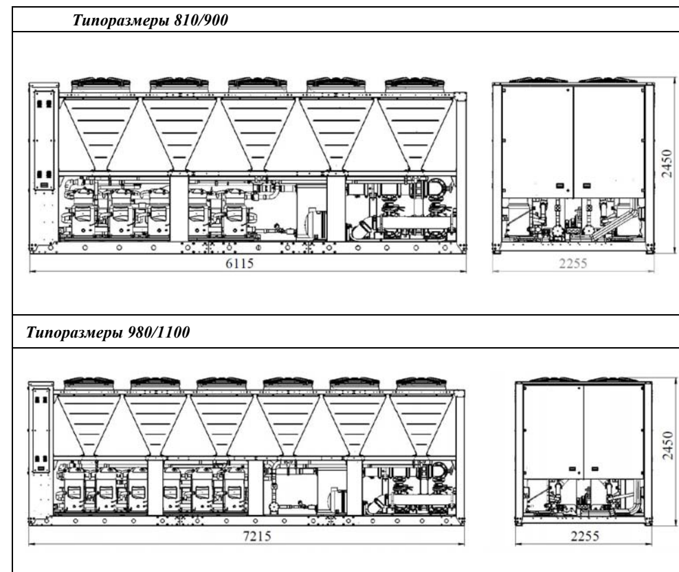
Рисунок 3.4. Основные размеры чиллеров типоразмеров 810-1100
