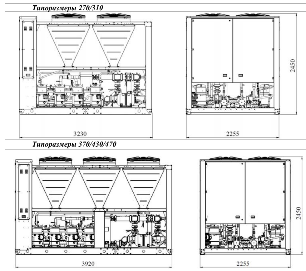
Рисунок 3.2. Основные размеры чиллеров 270-470
