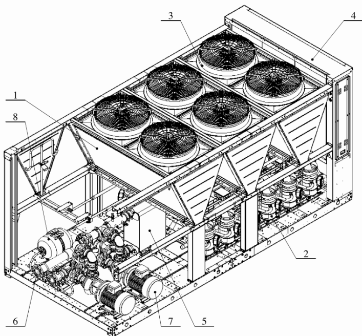
Рисунок 3.1. Компонировка чиллеров.
