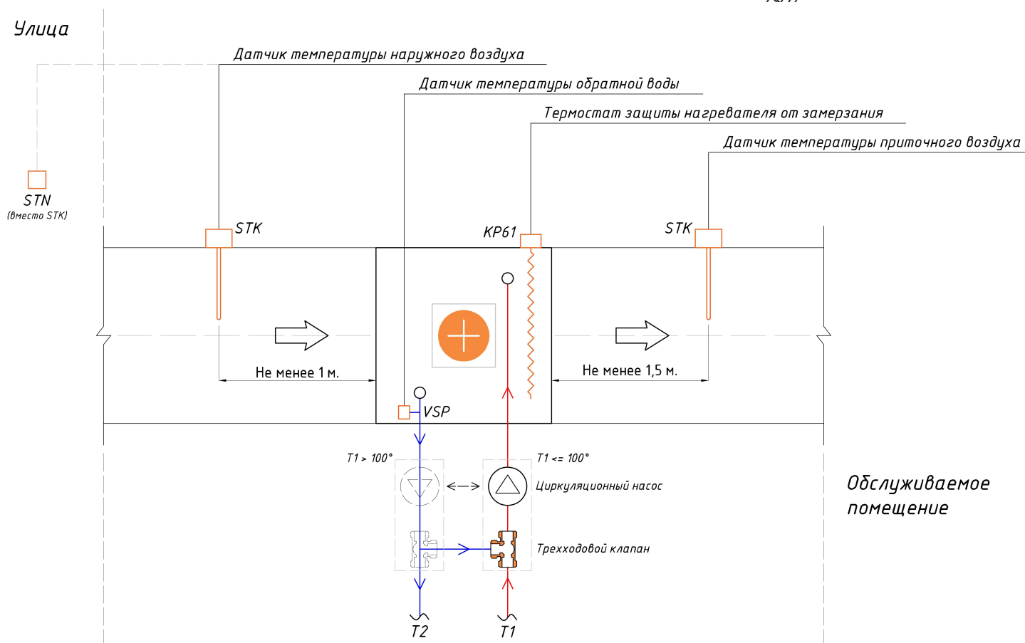
Рисунок 5.2 – Подключение датчиков
