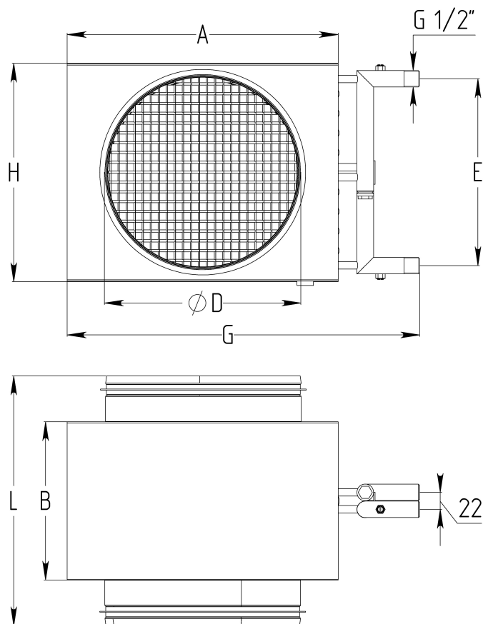
Рисунок 2.2 – Размеры воздухонагревателей
